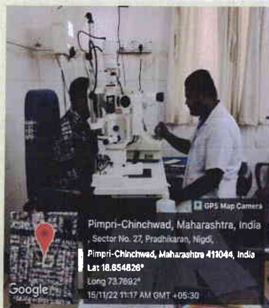
Autorefractometry
